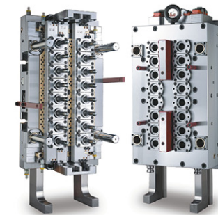
16腔瓶胚模具 16 Cavity Preform Mould
